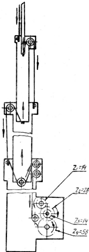
Рис. 11. Кинематическая схема телескопической мачты.
