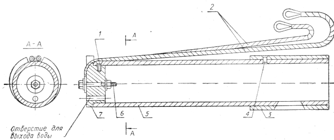
Рис. 4. Подвижное колено мачты: 1 — винт; 2 — двойной трос; 3 — бандажное кольцо; 4 — заклепка; 5 — труба; 6 — болт; 7 — основание.
